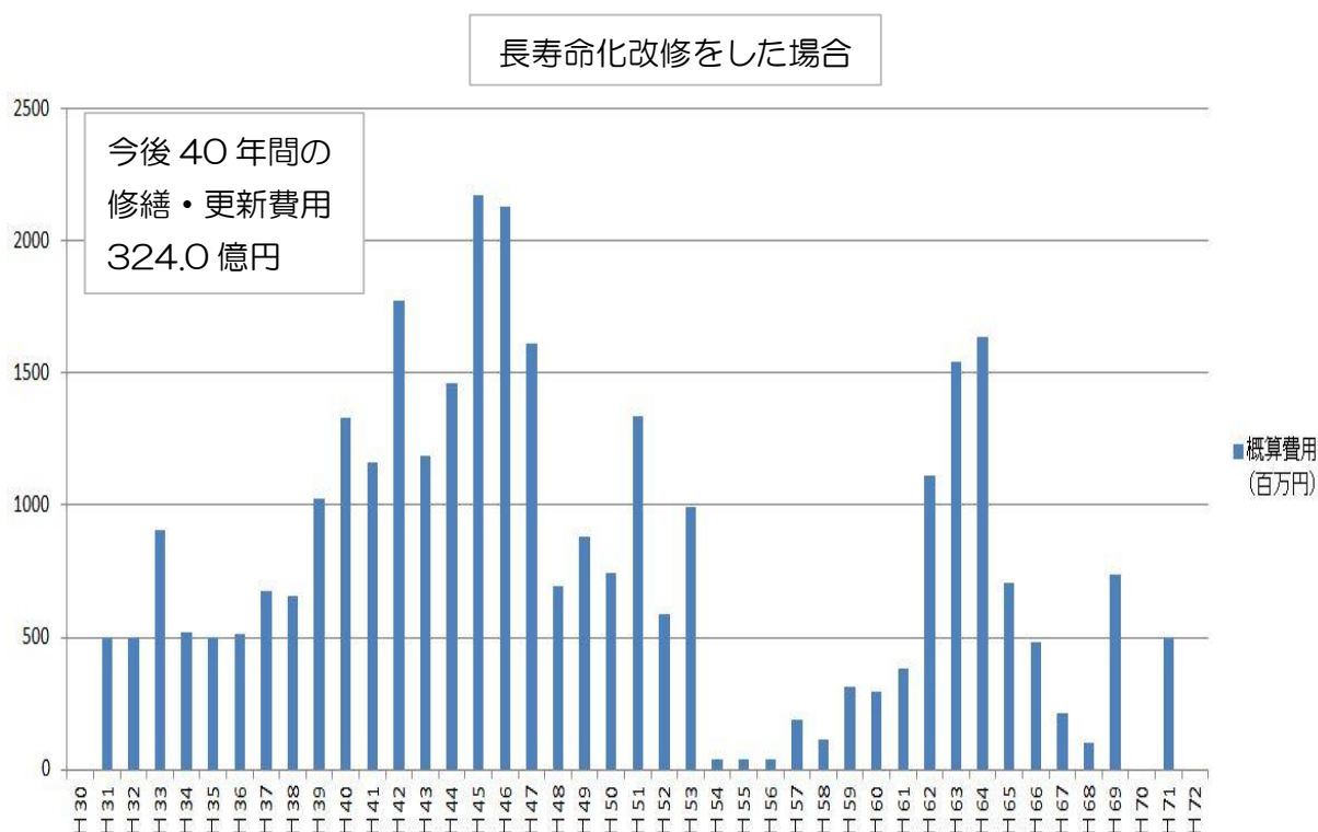
今後40年の修繕、更新費用試算 (図3)
